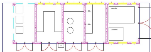
* Esquema simplificado da planta baixa da ATT em AutoCad.
